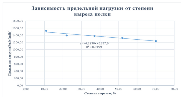
Рисунок 4. Зависимость предельной нагрузки от степени выреза полки P_{u,def} = f(\alpha)
