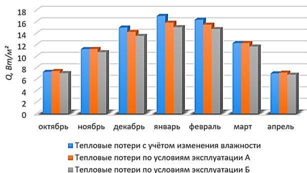
Рисунок 2 – Тепловые потери для ограждающей конструкции панельного здания с утеплителем ТЕХНОФАС ПРОФ
