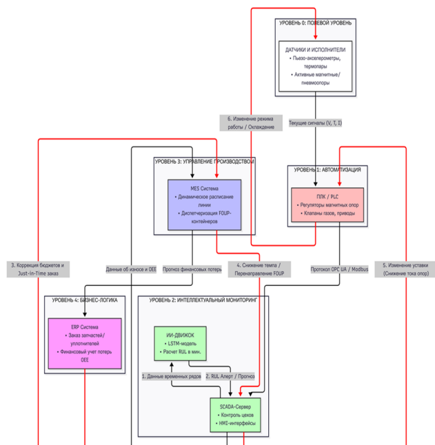
Рис. 1 Концептуальная схема метода интеграции предиктивного интеллектуального мониторинга в структуру действующей СМК предприятия в соответствии с требованиями разделов 6.1, 7.1.3 и 9.1 стандарта ГОСТ Р ИСО 9001-2015
