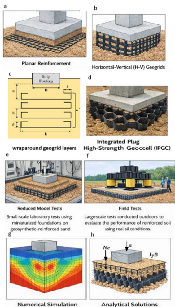
Рис. 1. Методы армирования оснований и подходы к их исследованию
