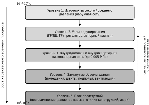
Рис. 1. Структурная схема динамической декомпозиции газовой системы жилой застройки
