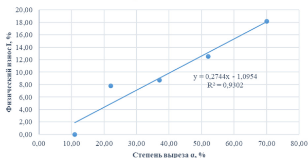
Рисунок 3. Зависимость физического износа от степени выреза полки I = f(\alpha)
