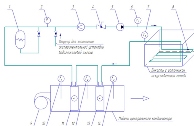
1 – гидроаккумулятор; 2 – манометр; 3 – преобразователь расхода электромагнитный; 4 – клапан балансировочный ручной; 5 – насос циркуляционный; 6, 7, 10, 12, 14 – термопреобразователи сопротивления; 8 – теплообменник источника естественного холода; 9 – вентилятор модели центрального кондиционера; 11, 13 – водо-воздушные теплообменники блока воздухоохладителя 1-й и 2-й ступеней модели Рис. 1 – Принципиальная схема установки [2]
