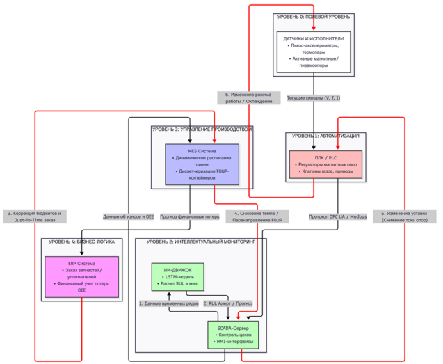
Рис. 1 Концептуальная схема метода интеграции предиктивного мониторинга процессов литографии в структуру CMK [1]
