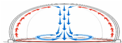
Рис. 2. Аэродинамическая схема тороидального свободно-конвективного течения в объеме РПУ
