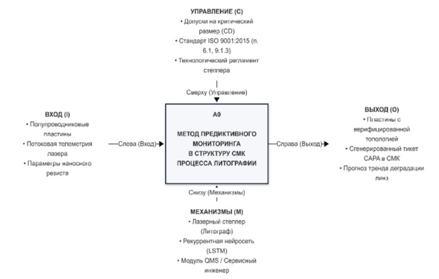
Рис. 2 Функциональная структура метода интеграции предиктивного мониторинга процессов литографии в структуру CMK в нотации IDEF0 (A0)
