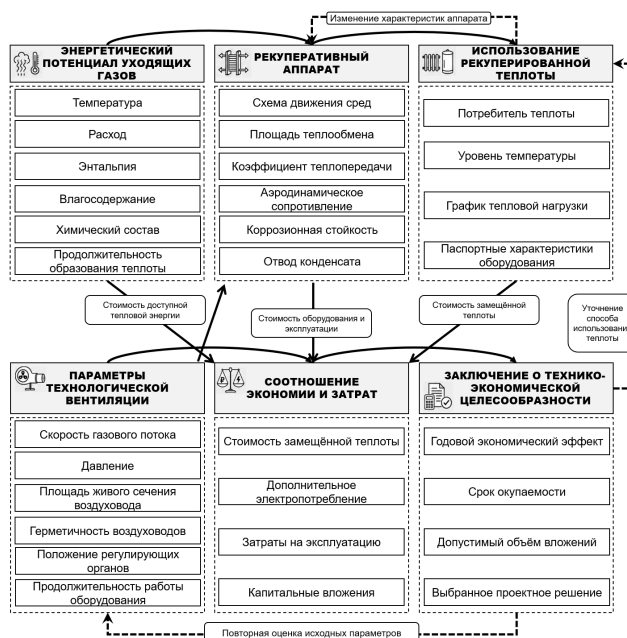
Рисунок 1 – Обобщённая модель стратегии технико-экономического обоснования рекуперации теплоты в системе технологической вентиляции здания Источник: авторская разработка
