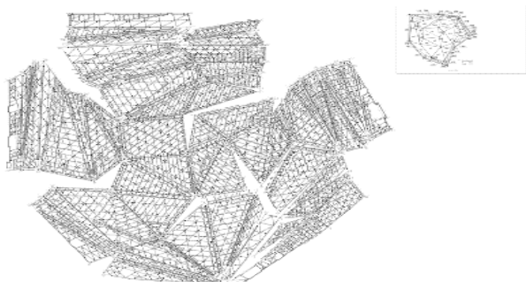
Рис.3 Оперный театр в Гуанчжоу, развернутый макет основной стальной конструкции.
